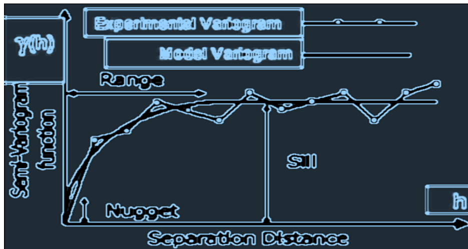
Fig. 4. Parameters of semi-variogram
